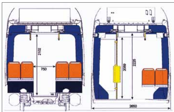
Vagnsbredden 2,65 meter möjliggör naturligtvis generösa innerutrymmen, med bland annat fri bredd i mittgång på ca 700 mm. Väljer man smalare sittplatser kan mittgångsbredd ökas till ca 750 mm, som på bilden. Ritning: Bombardier Transportation
